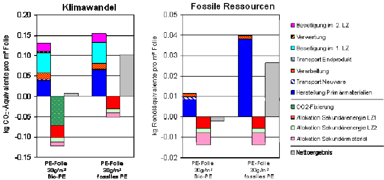
Abbildung 14: Ökobilanzieller Vergleich von Folienverpackungen aus fossilem PE und Bio-PE (Ergebnisse für den Indikator Klimawandel und fossiler Ressourcenverbrauch)
