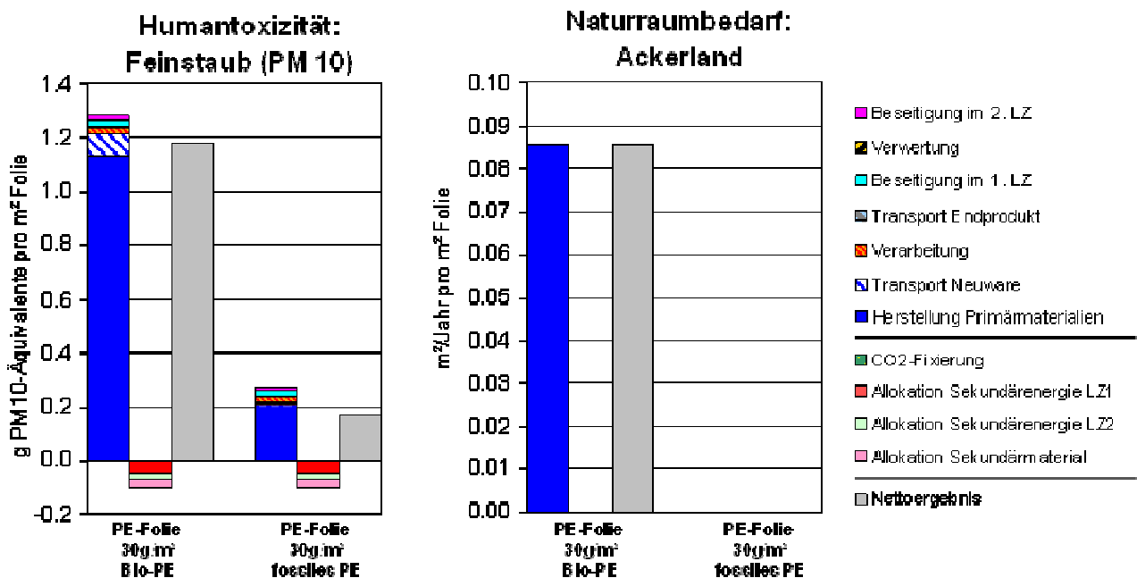
Abbildung 17: Ökobilanzieller Vergleich von Folienverpackungen aus fossilem PE und Bio-PE (Ergebnisse für den Indikator Humantoxizität: Feinstaub [PM10] und Naturraumbeanspruchung: Ackerland)
