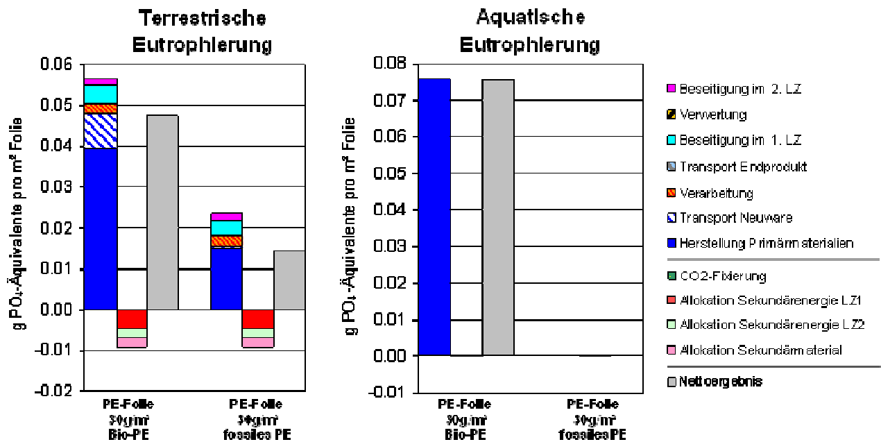
Abbildung 16: Ökobilanzieller Vergleich von Folienverpackungen aus fossilem PE und Bio-PE (Ergebnisse für den Indikator terrestrische und aquatische Eutrophierung)
