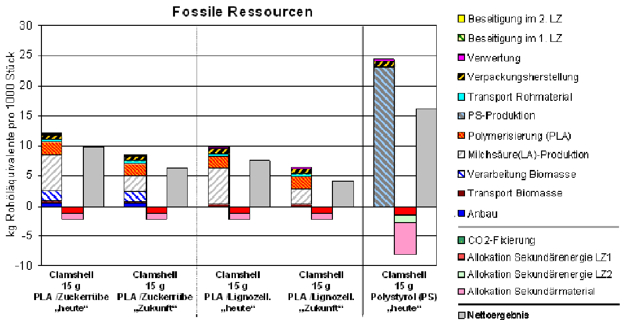
Abbildung 20: Ökobilanzieller Vergleich von Klappdeckelschalen aus PLA und PS (Ergebnisse für den Indikator fossiler Ressourcenverbrauch)
