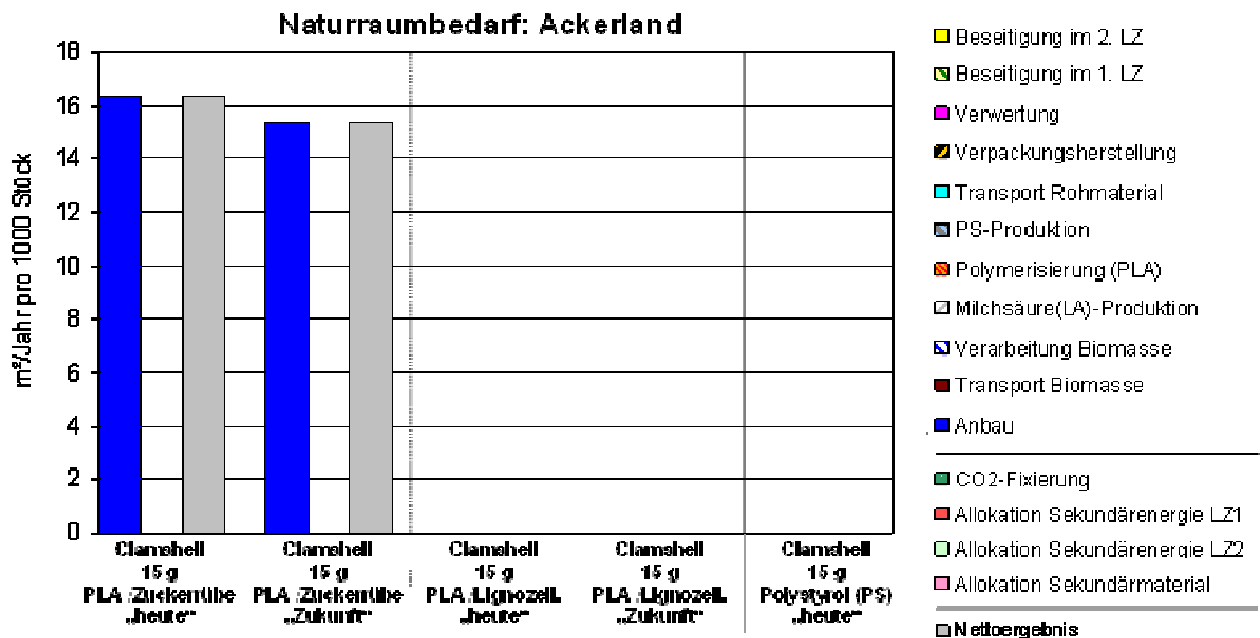
Abbildung 26: Ökobilanzieller Vergleich von Klappdeckelschalen aus PLA und PS (Ergebnisse für den Indikator Naturraumbanspruchung: Ackerland)
